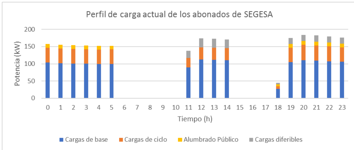
Ilustración 11: Perfil de carga basado en los registros de 6 al 8 de noviembre 2018
