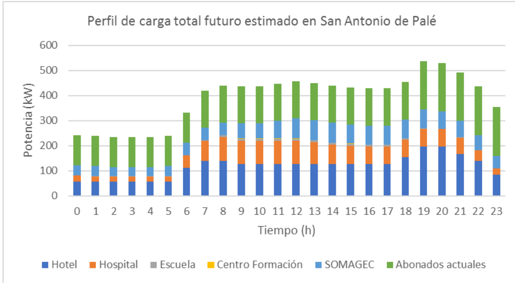
Ilustración 27: Perfil de carga total futuro en San Antonio de Palé
