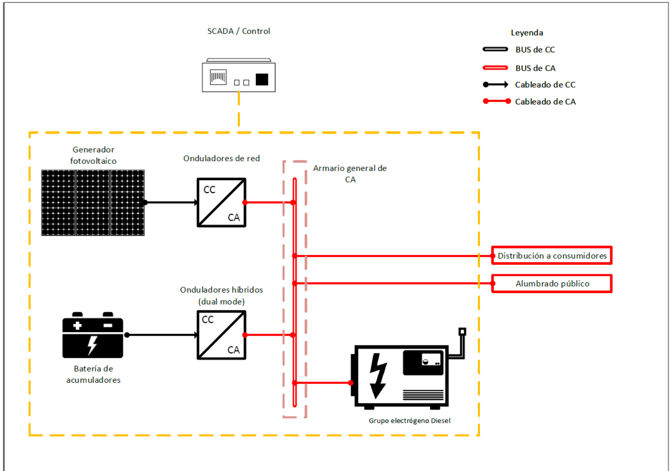
Ilustración 45: Diagrama Unifilar de la planta
