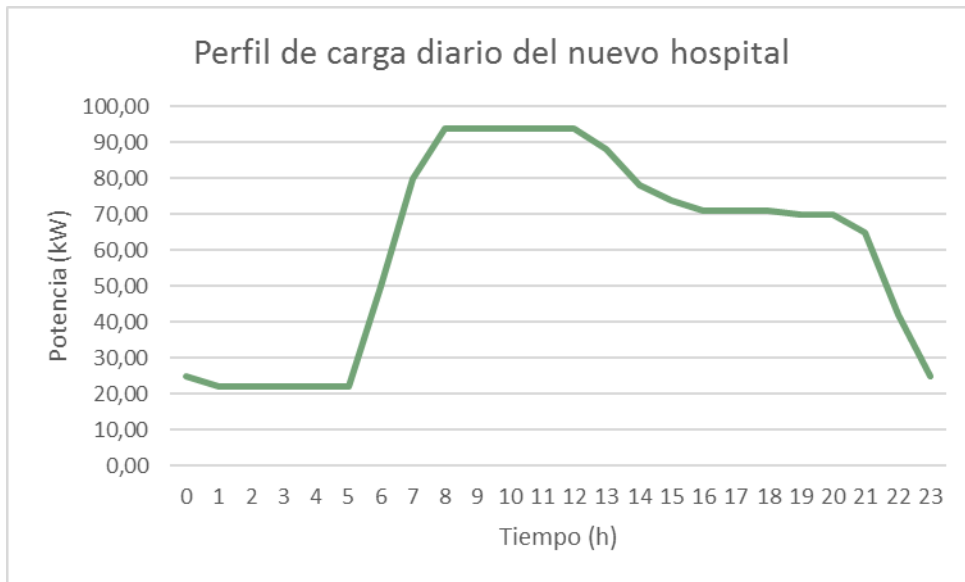
Ilustración 24: Perfil de carga diario para el nuevo hospital de San Antonio de Palé
