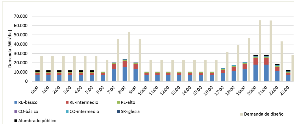
Ilustración 32: Perfil de carga desglosado en año 1 y perfil de demanda de diseño en año 5 en Awal
